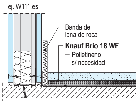
F126.es-V1 Encuentro con tabique en zona húmeda
